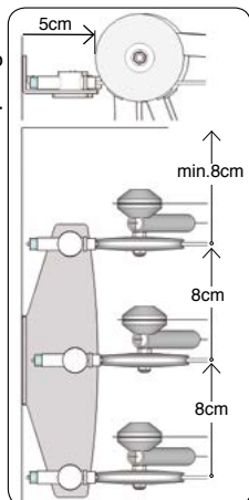
Wandbefestigung dreiläufig/ wall bracket 3 tracks
