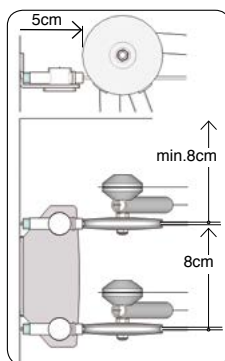
Wandbefestigung zweiläufig/ wall bracket two tracks
