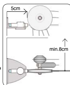
Wandbefestigung einläufig/ wall bracket one track
