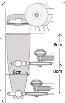
Wandwinkel zweiläufig/ wall angle two tracks
