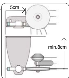
Wandwinkel einläufig/ wall angle one track
